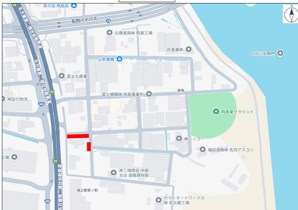
工事箇所図
